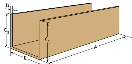
U-Profil
