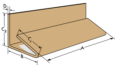
U-Profil mit Klemmeffekt
